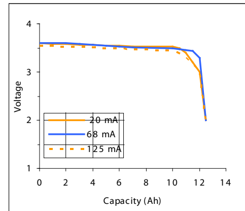
150°C discharge
